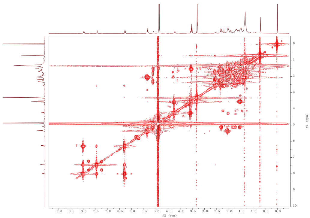
图 21 化合物 2 的 ^1\text{H} - ^1\text{H} COSY 图谱
