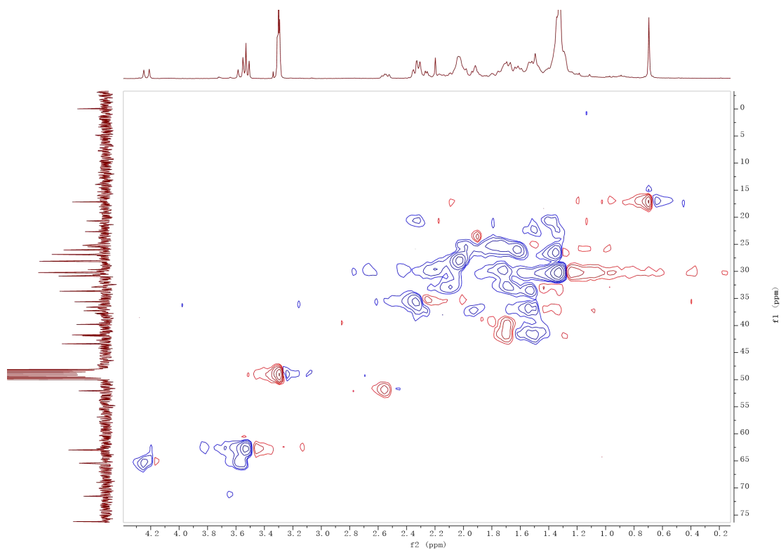
图 23 化合物 2 的放大 HSQC 图谱
