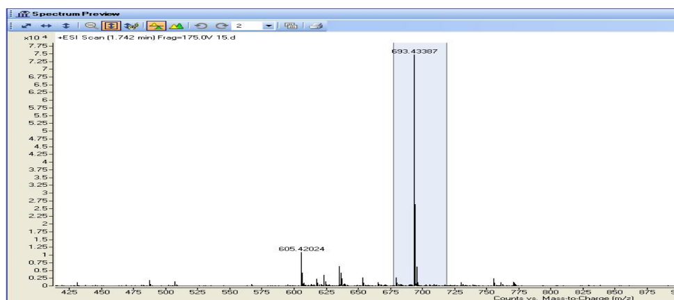
图 18 化合物 2 的 HR-ESI-MS 图谱
