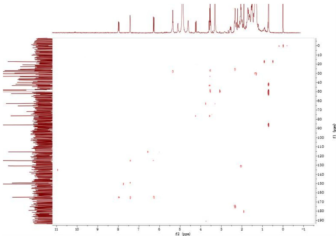
图 8 化合物 1 的 HMBC 图谱
