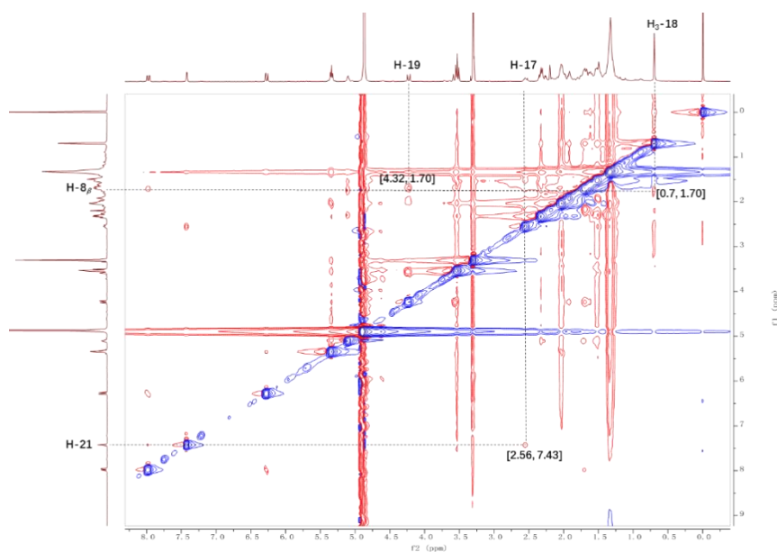
图 13 化合物 1 的关键 NOESY 信号
