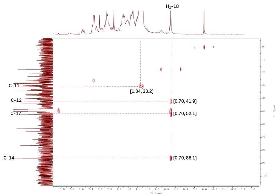
图 9 化合物 1 的关键 HMBC 信号
