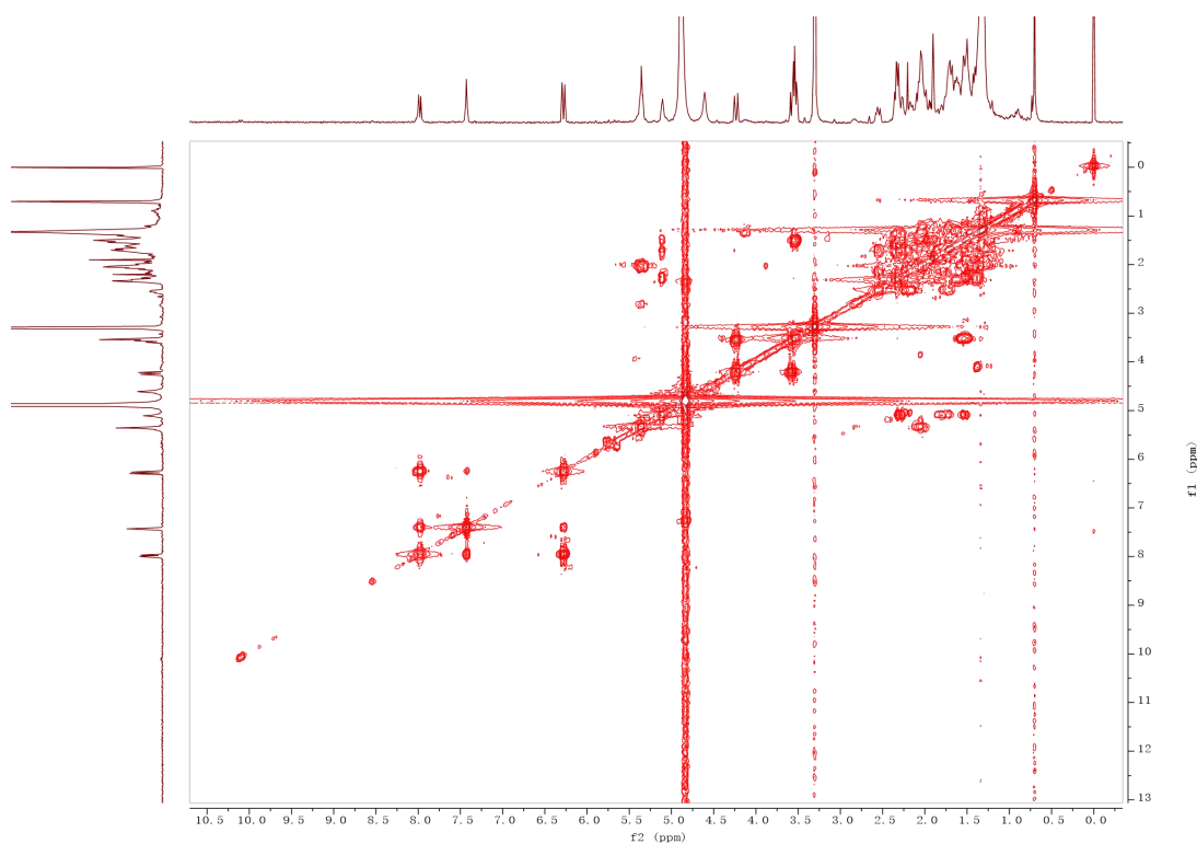
图 5 化合物 1 的 ^1\text{H} - ^1\text{H} COSY 图谱
