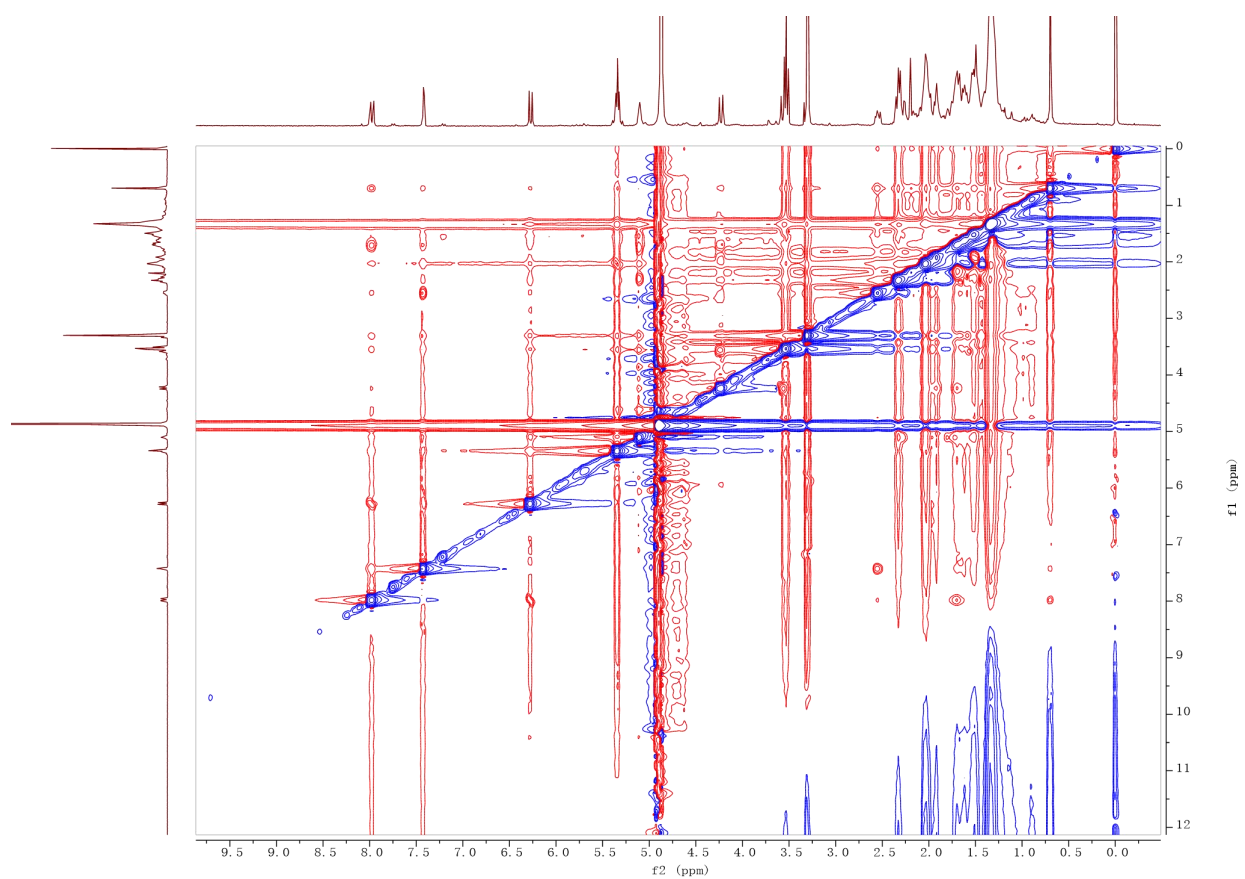
图 27 化合物 2 的 NOESY 图谱
