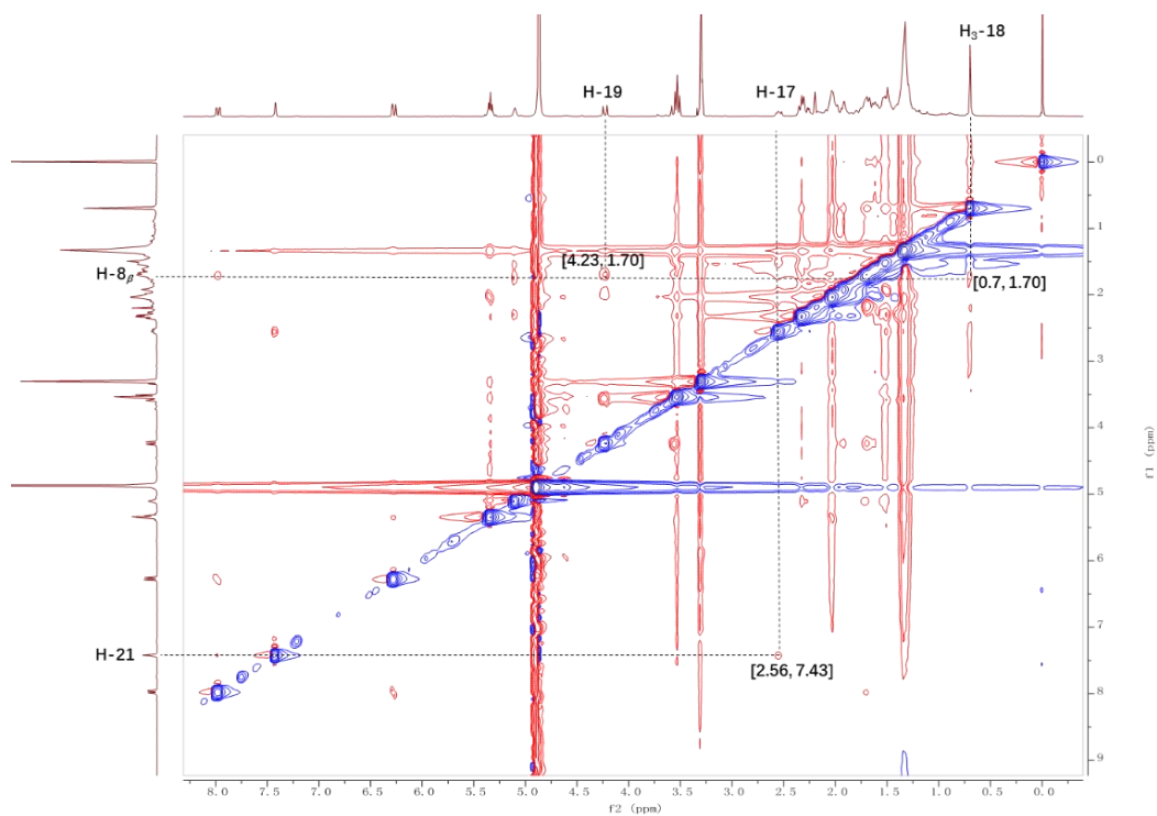
图 29 化合物 2 的放大 NOESY 图谱
