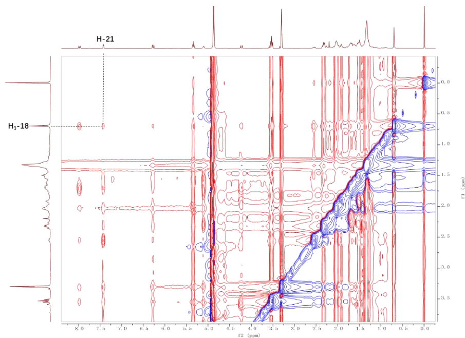
图 14 化合物 1 的关键 NOESY 信号
