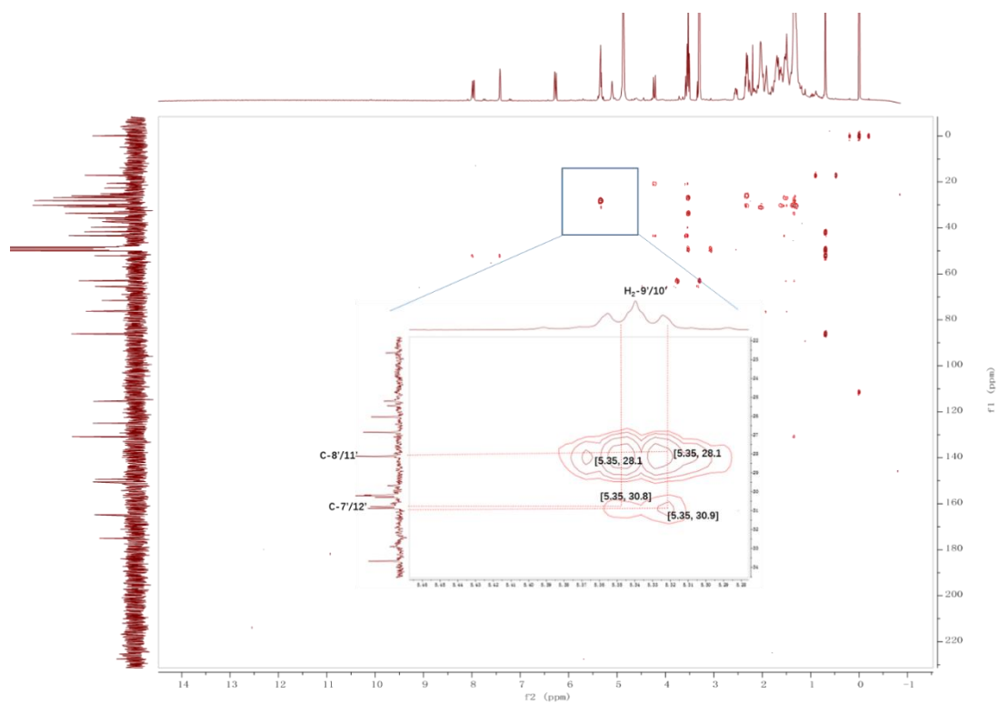
图 26 化合物 2 的关键 HMBC 信号
