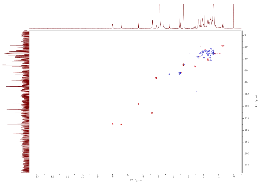
图 6 化合物 1 的 HSQC 图谱
