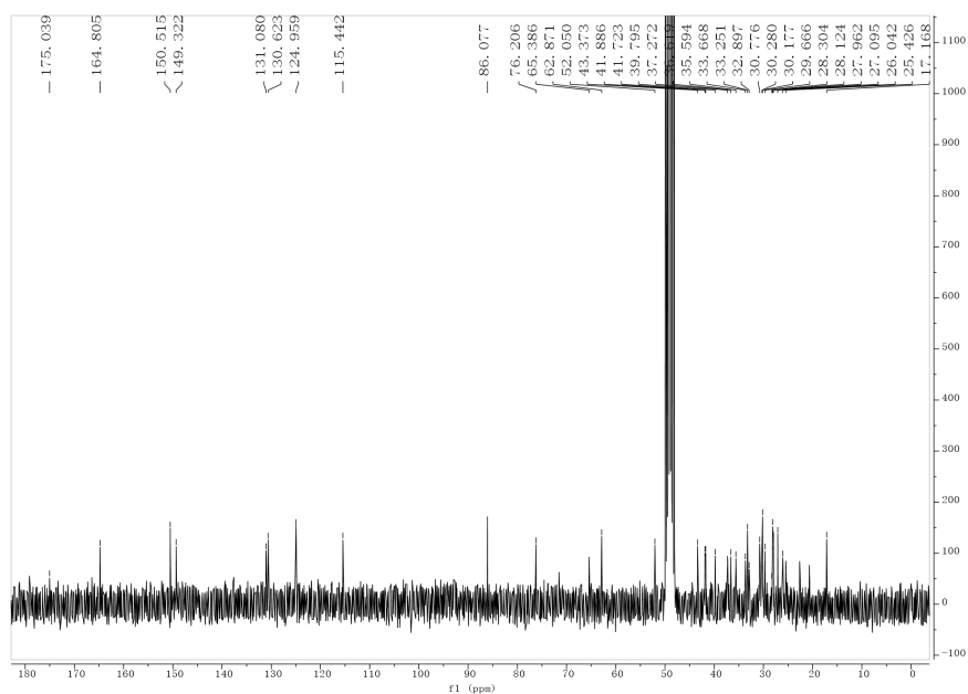
图 4 化合物 1 的 ^{13}\text{C} NMR 图谱
