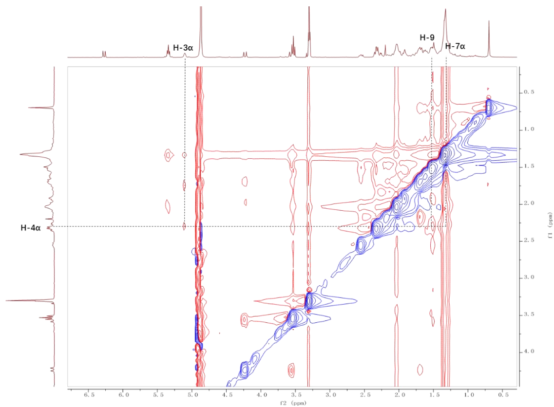
图 28 化合物 2 的放大 NOESY 图谱
