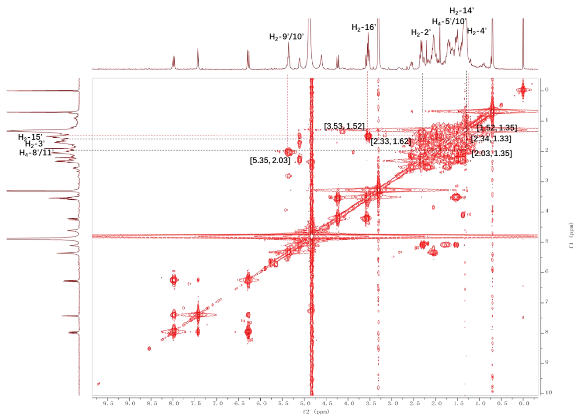
图 24 化合物 2 的关键 ^1\text{H} - ^1\text{H} COSY 信号
