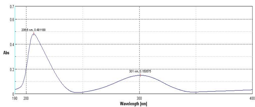
图 17 化合物 2 的 UV 图谱
