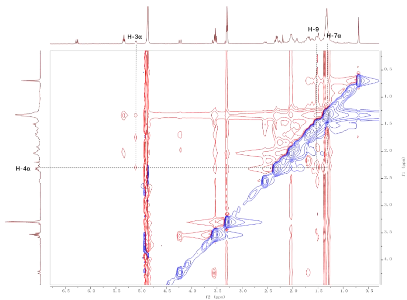
图 12 化合物 1 的关键 NOESY 信号
