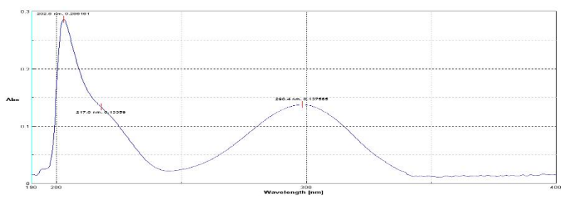
图 1 化合物 1 的 UV 图谱
