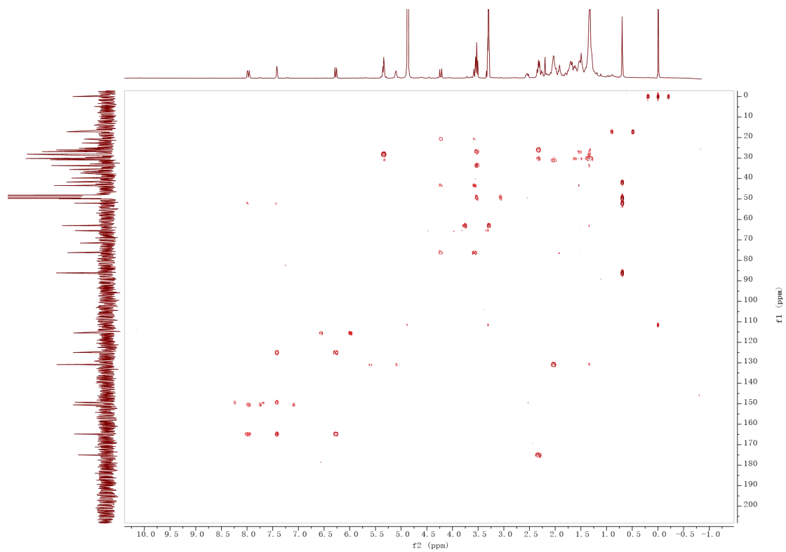
图 25 化合物 2 的 HMBC 图谱
