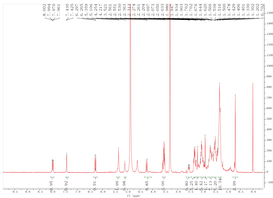
图 3 化合物 1 的 1 H NMR 图谱
