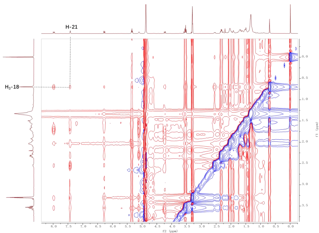
图 30 化合物 2 的放大 NOESY 图谱
