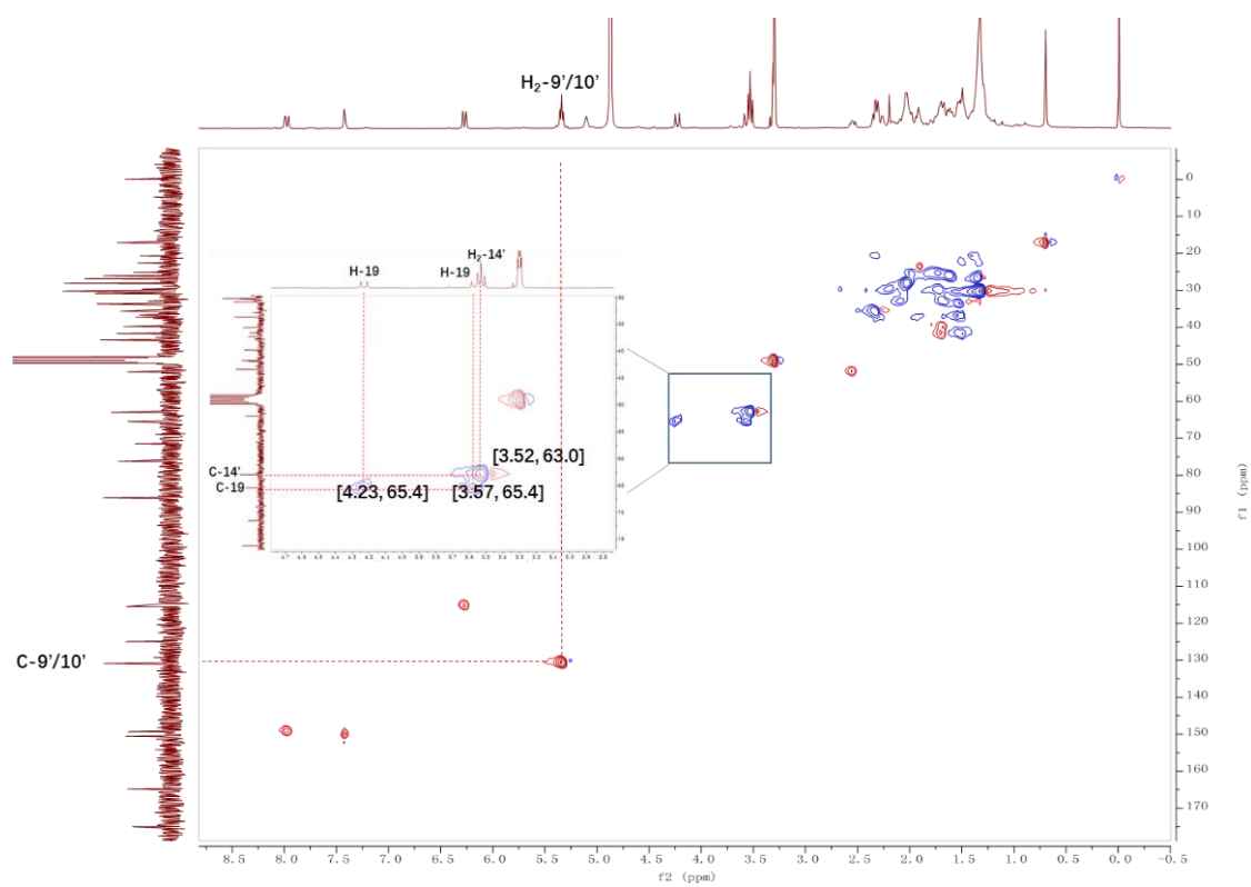
图 22 化合物 2 的 HSQC 图谱
