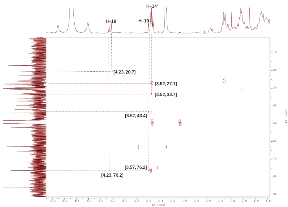
图 10 化合物 1 的关键 HMBC 信号
