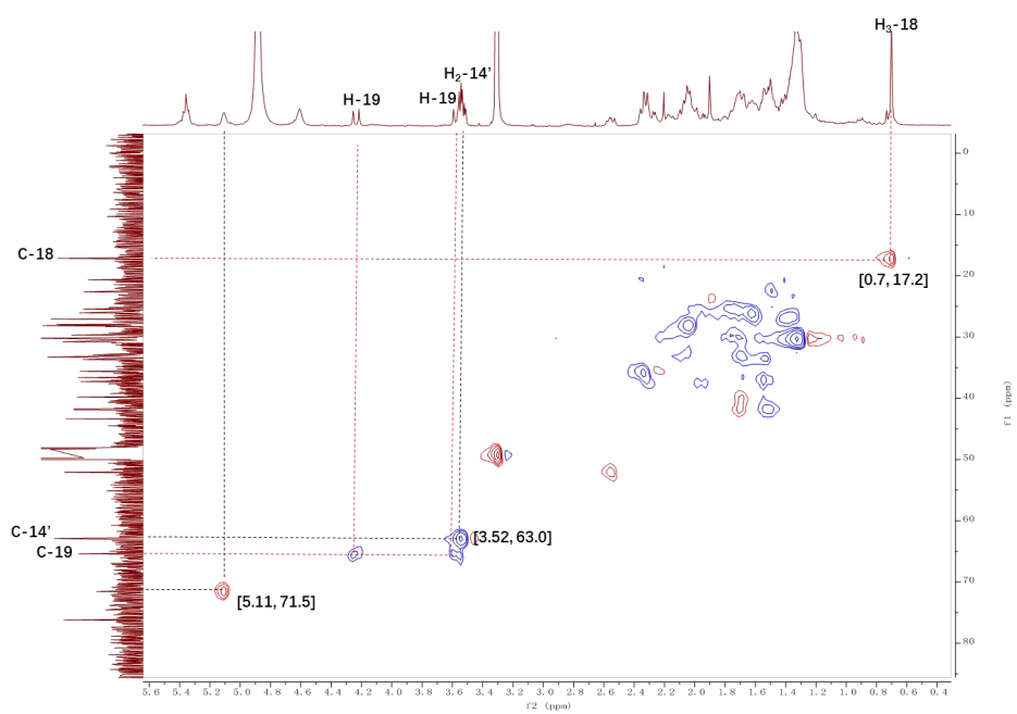
图 7 化合物 1 的关键 HSQC 相关信号
