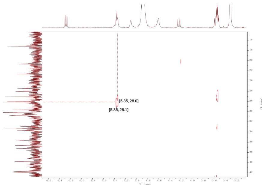
图 16 化合物 1 的关键 HMBC 信号
