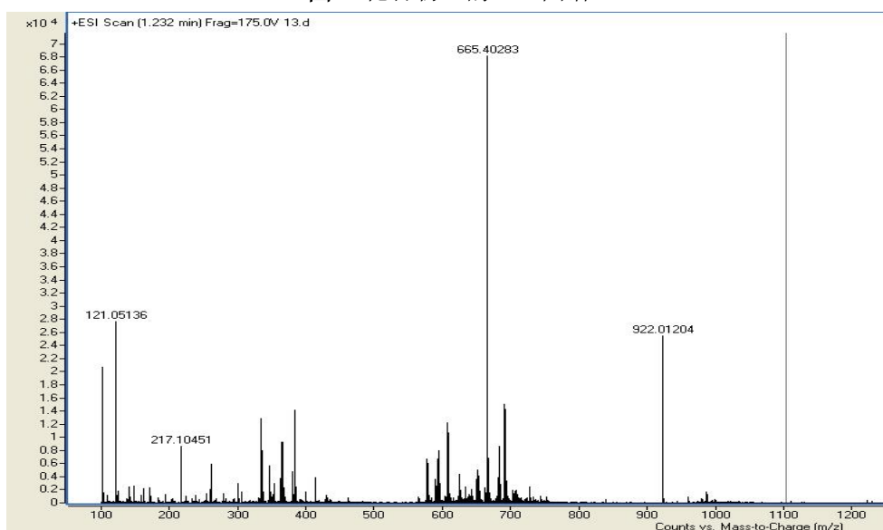
图 2 化合物 1 的 HR-ESI-MS 图谱
