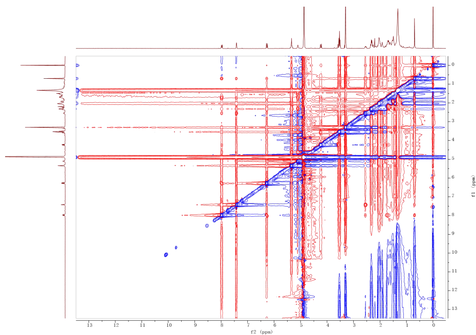
图 11 化合物 1 的 NOESY 图谱
