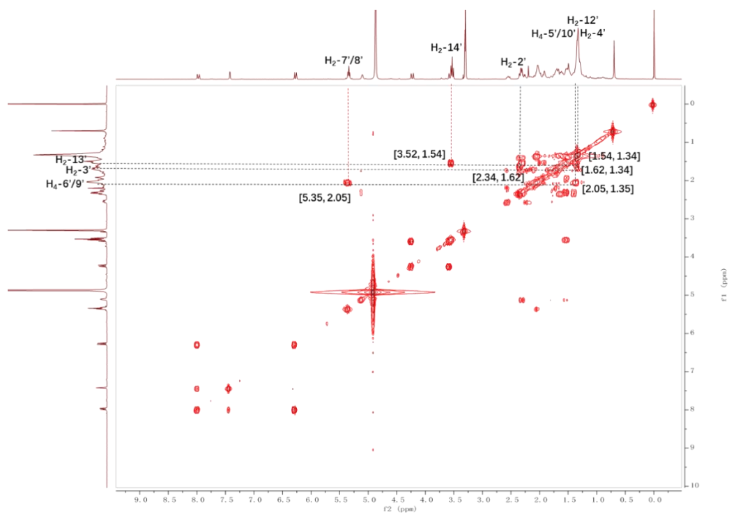
图 15 化合物 1 的关键 1 H- 1 H COSY 信号
