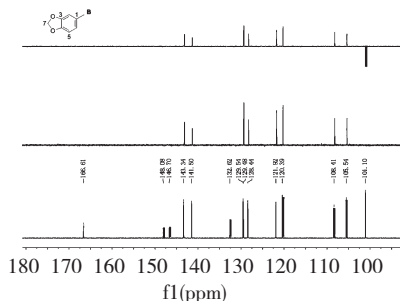
图 3 以化合物 1 为例 A 片段的碳谱及 DEPT 谱信号特征(加粗标出部分)
