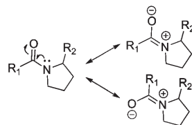
图11 吡咯类酰胺生物碱的结构特征
