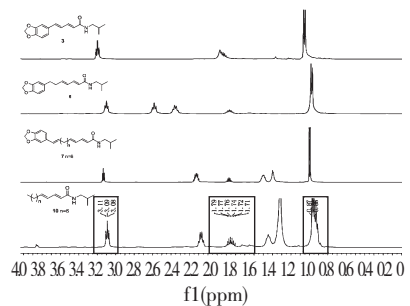
图 13 酰胺生物碱 C2 片段的氢谱的信号特征 (方框部分)
