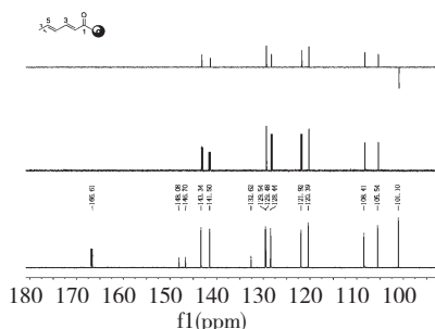
图 5 以化合物 3 为例 B2 片段的碳谱及 DEPT 谱信号特征(加粗标出部分)
