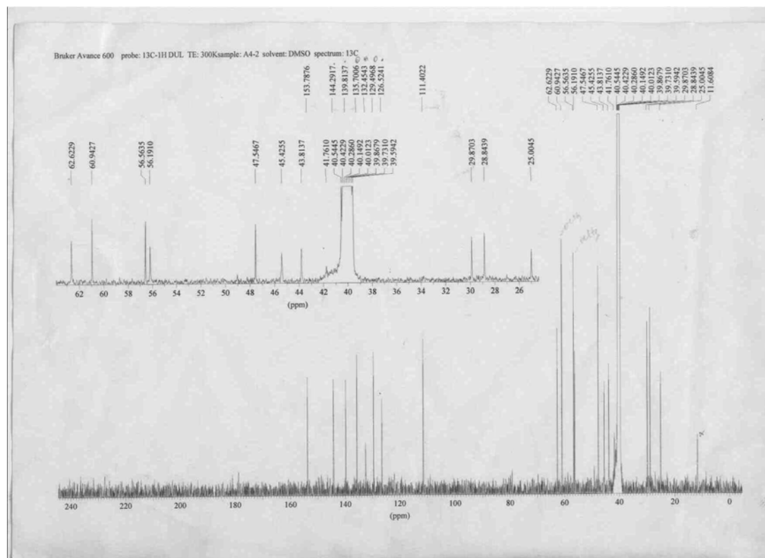
图 1 化合物 1 的 13 C-NMR 谱
