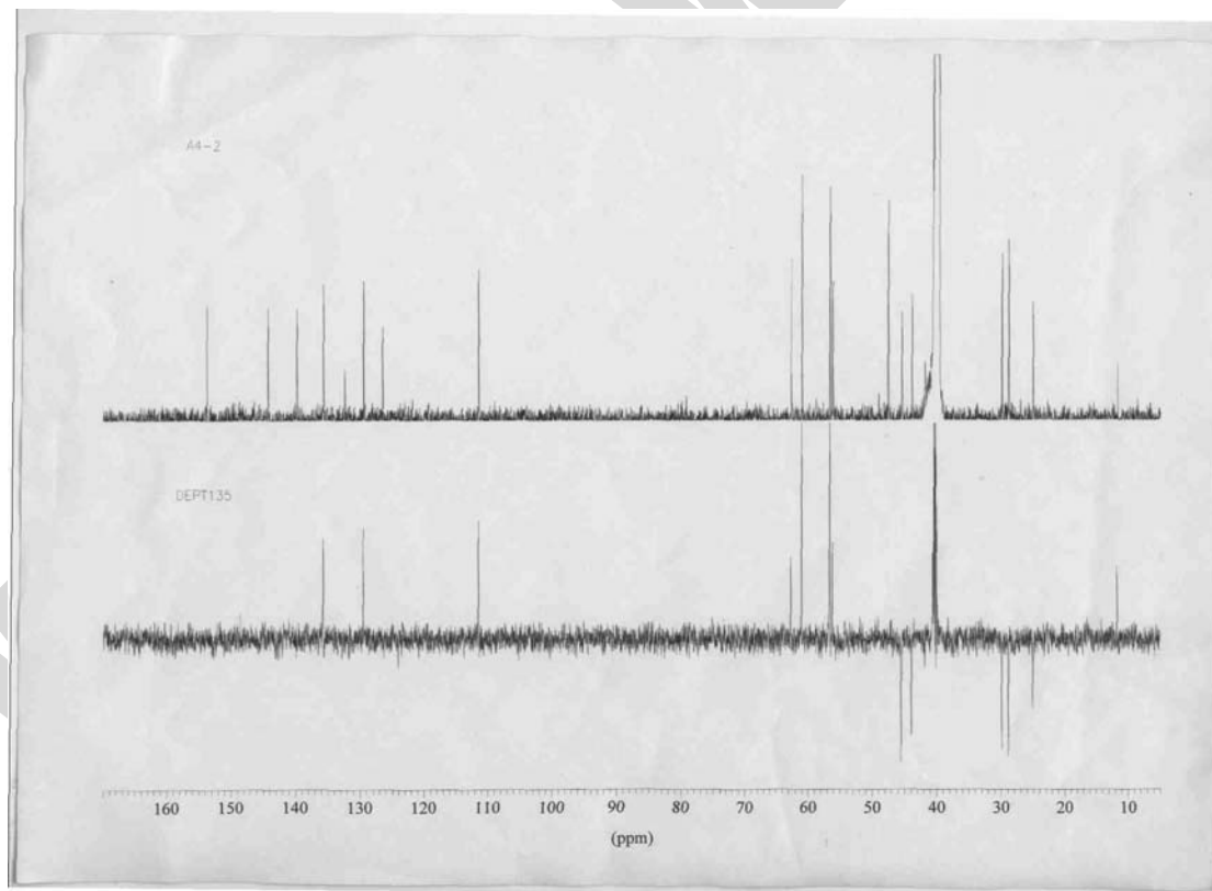
图 3 化合物 1 的 DEPT 谱
