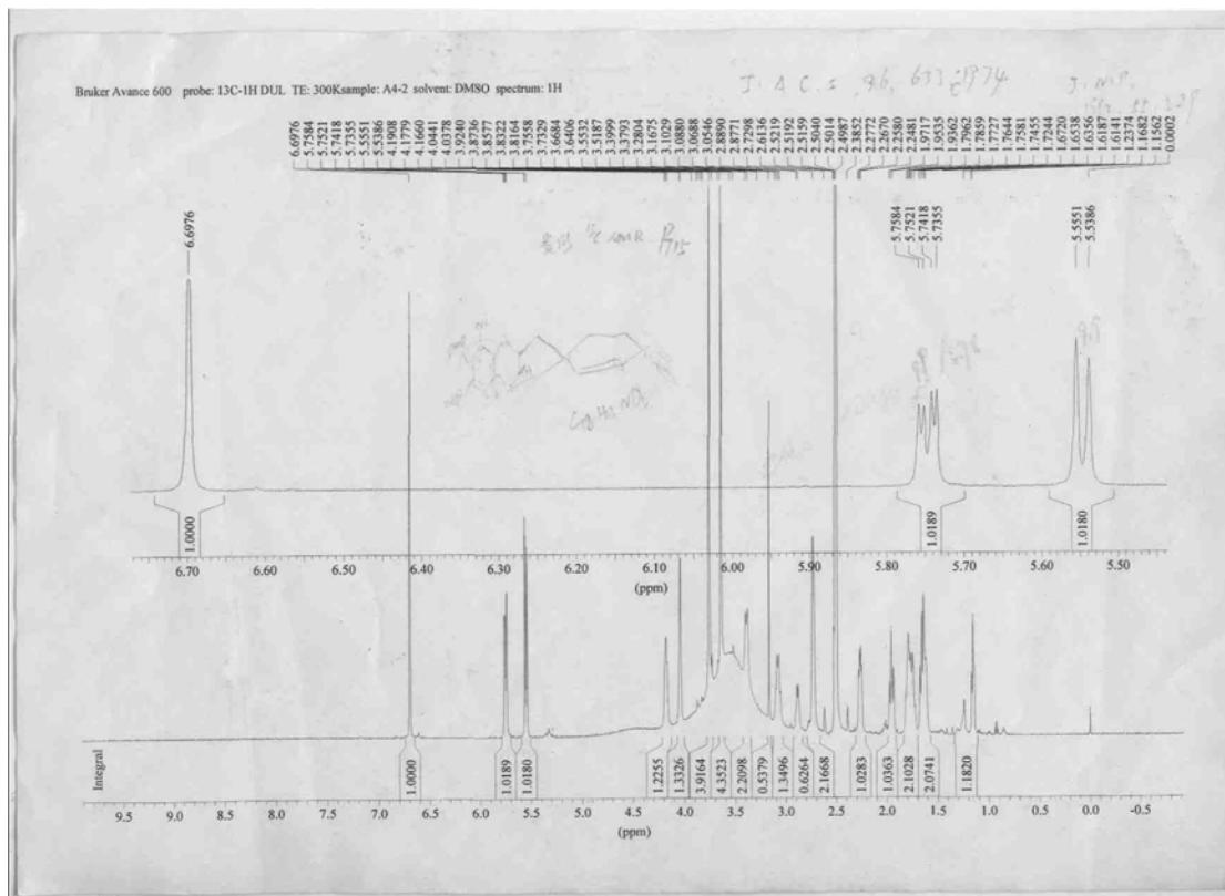
图 2 化合物 1 的 ^1\text{H} -NMR 谱
