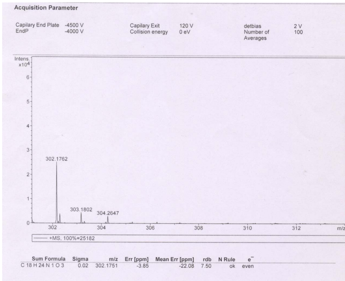
图 4 化合物 1 的高分辨质谱图
