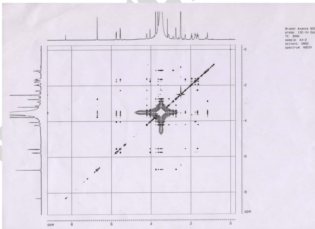
图 5 化合物 1 的 NOESY 图
