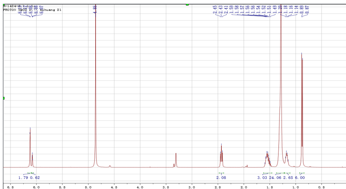
图 1 Adiposatin E (1) 的 ^1\text{H-NMR} 图谱
