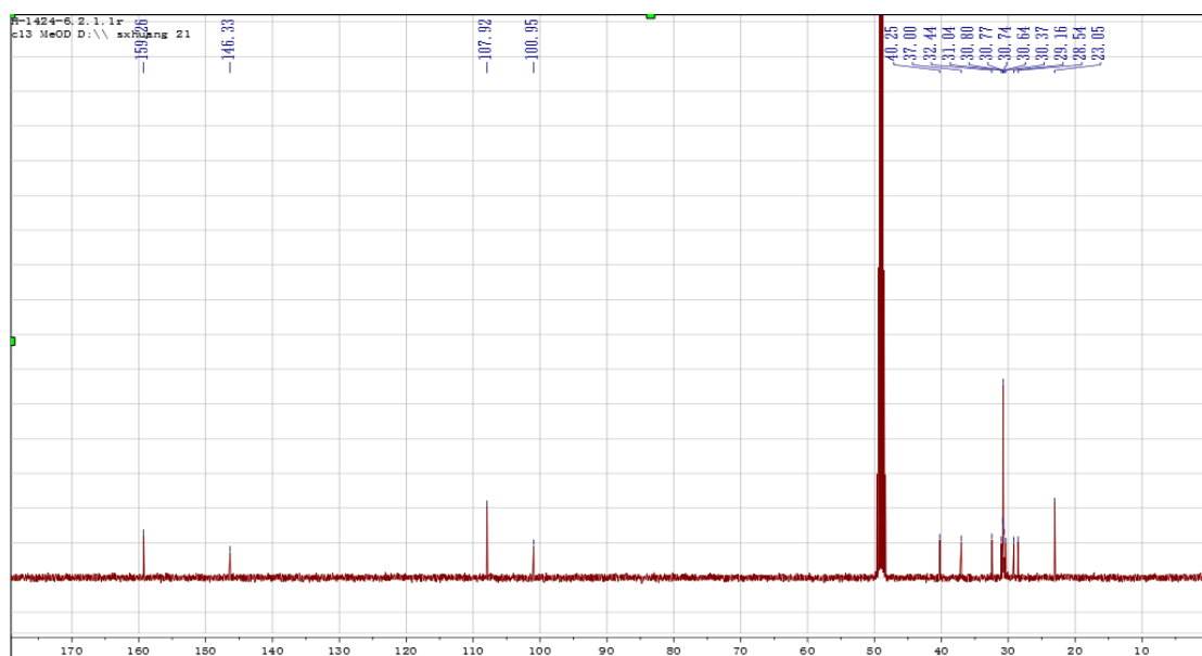
图 2 Adiposatin E (1) 的 ^{13}\text{C-NMR} 图谱
