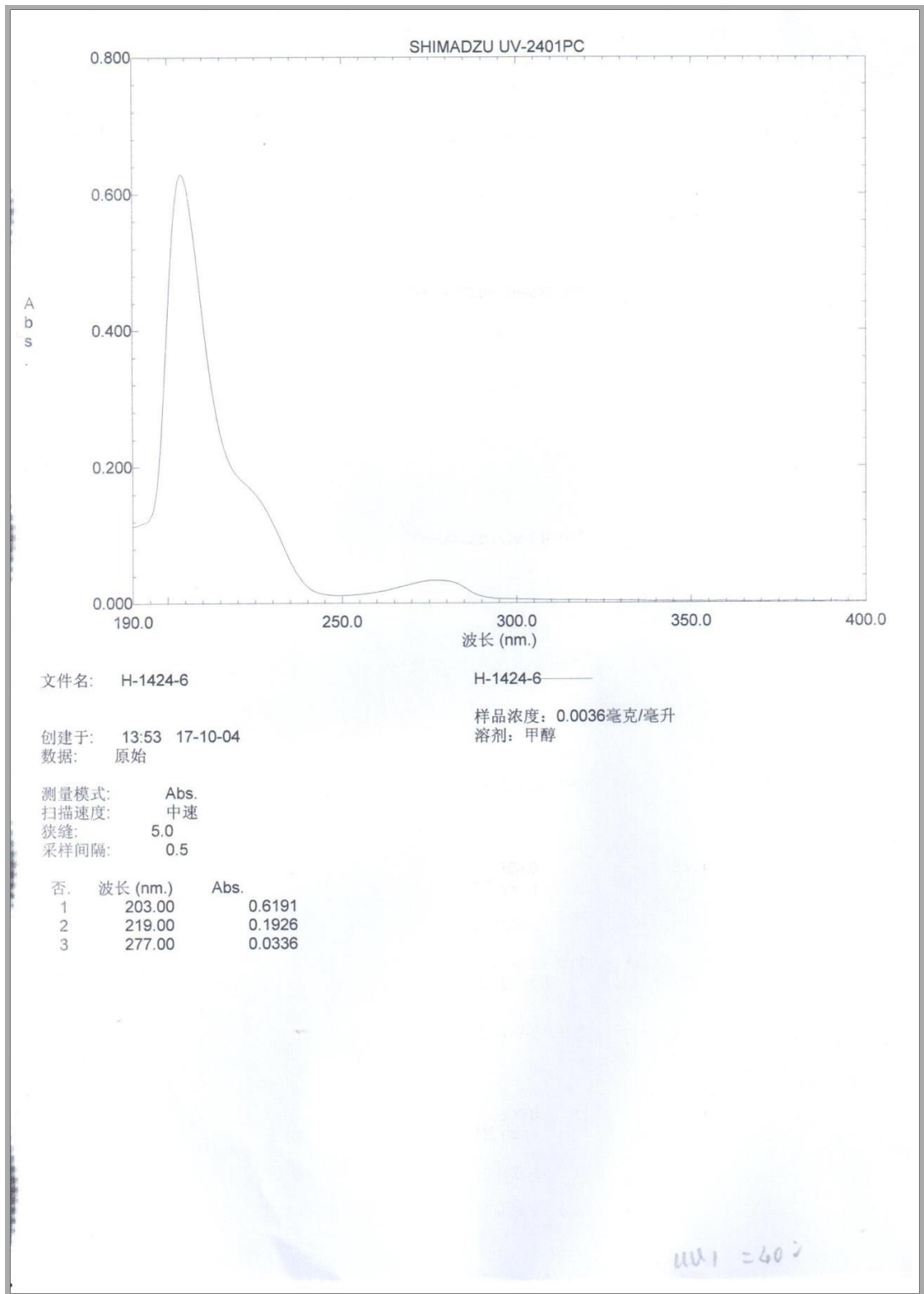
图 8 Adiposatin E (1) 的紫外图谱
