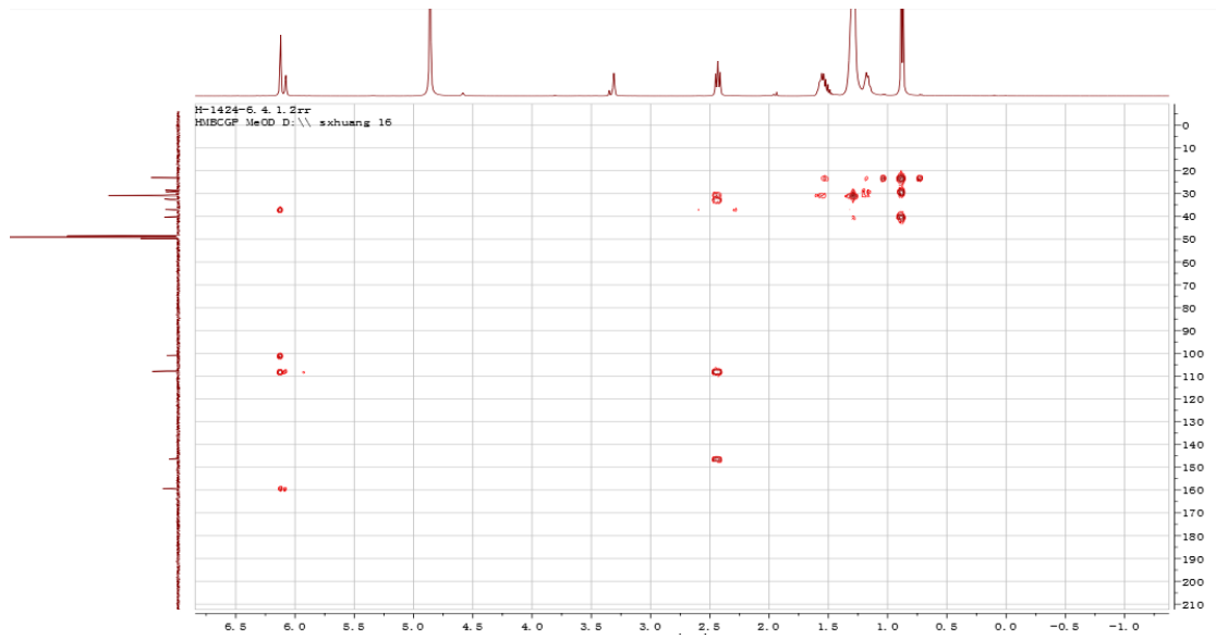
图3 Adiposatin E (1) 的 HSQC 图谱
