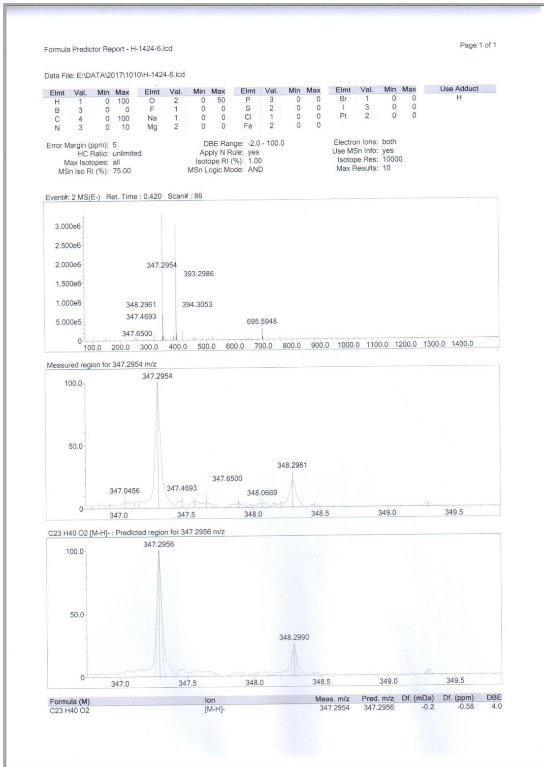
图 6 Adiposatin E (1) 的 HRESI 图谱
