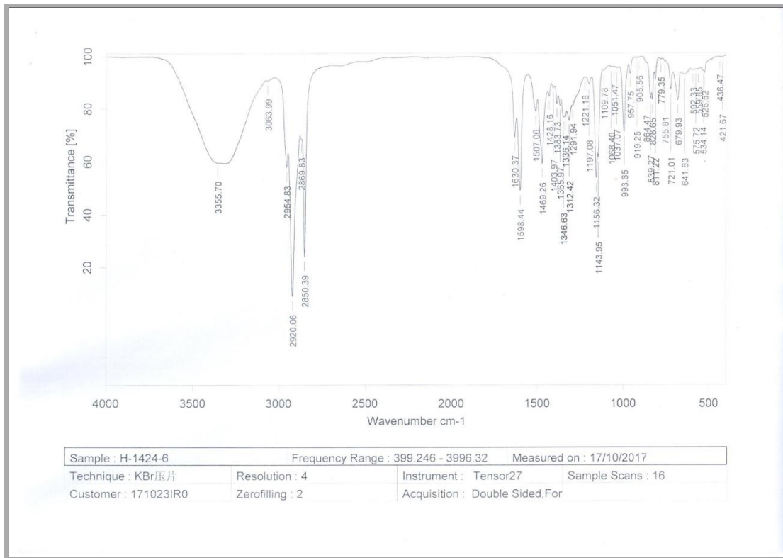
图 7 Adiposatin E (1) 的红外图谱
