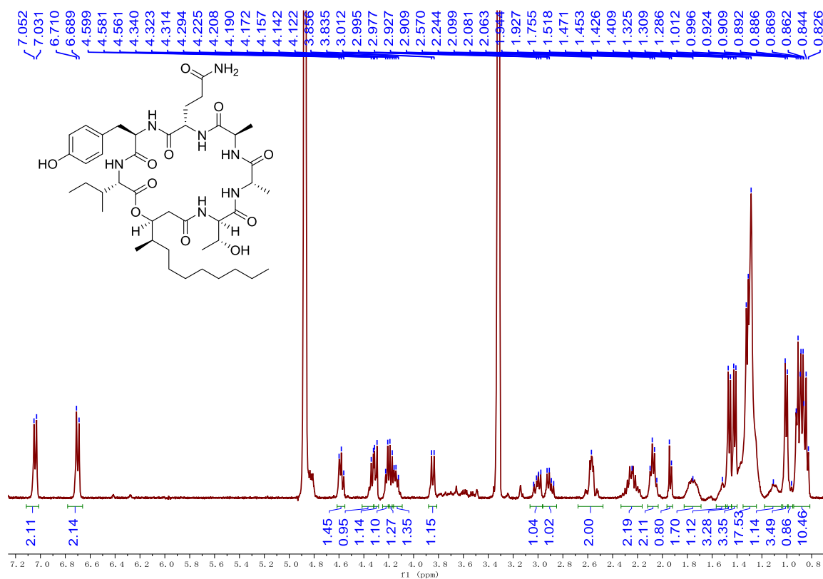
图 S6 化合物 1 的 ^1\text{H} NMR 谱
