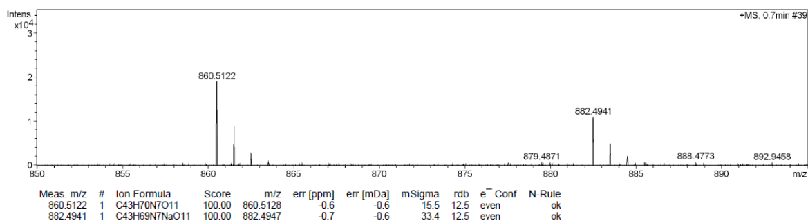
图 S11 化合物 1 的(+)-HR-ESI-MS 谱
