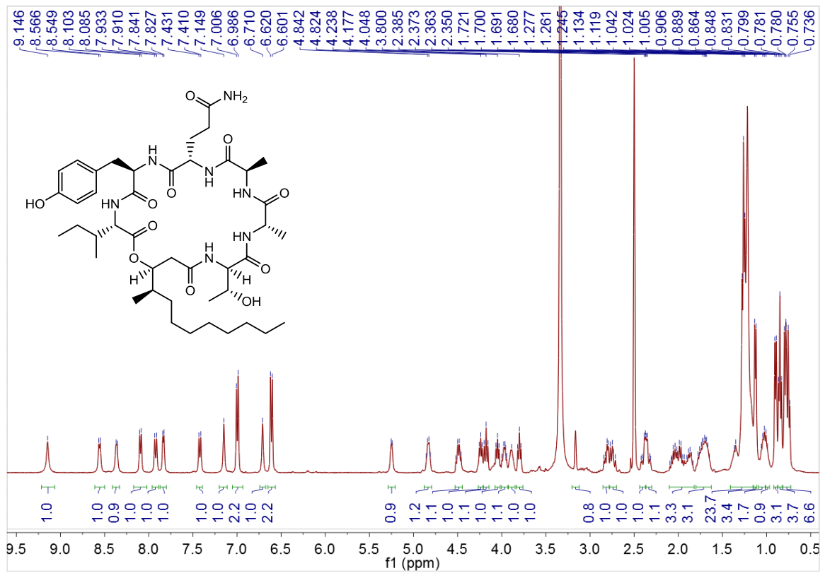
图 S1 化合物 1 的 ^1\text{H} NMR 谱 (DMSO- d_6 ) Figure S1. ^1\text{H} NMR spectrum of 1 in in DMSO- d_6
