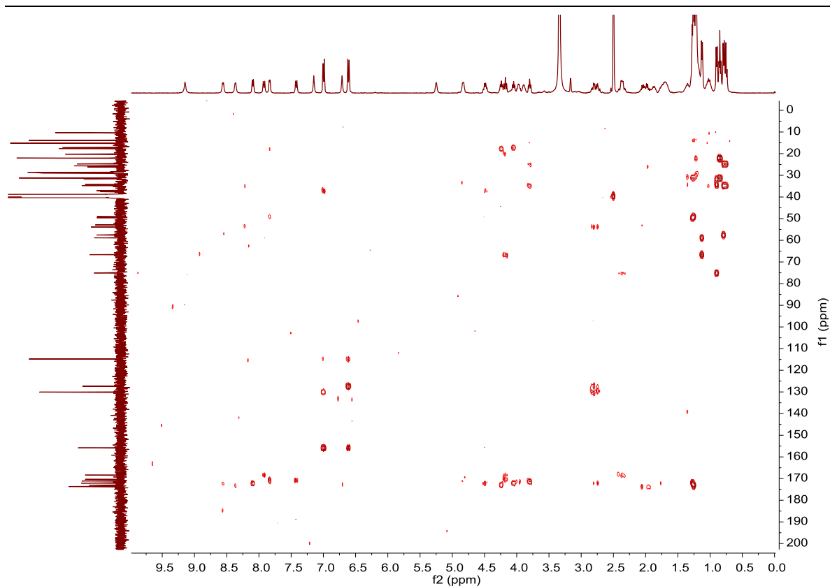
图 S5 化合物 1 的 HMBC 谱 (DMSO- d_6 )
