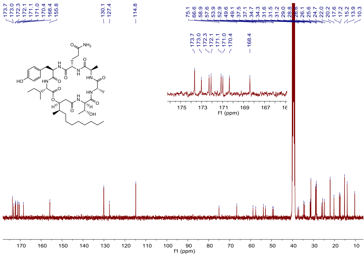
图 S2 化合物 1 的 ^{13}\text{C} NMR 谱 (DMSO- d_6 ) Figure S2. ^{13}\text{C} NMR spectrum of 1 in in DMSO- d_6
