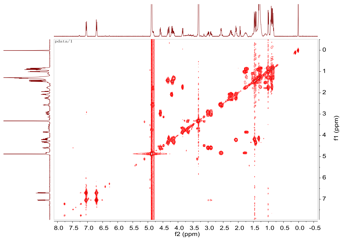
图 S8 化合物 1 的 ^1\text{H} - ^1\text{H} COSY 谱 ( \text{CD}_3\text{OD} ) Figure S8. ^1\text{H} - ^1\text{H} COSY NMR spectrum of 1 in \text{CD}_3\text{OD}
