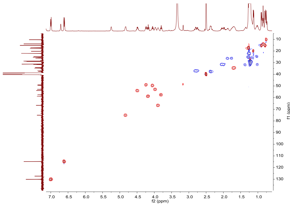
图 S4 化合物 1 的 HSQC 谱 (DMSO- d_6 )
