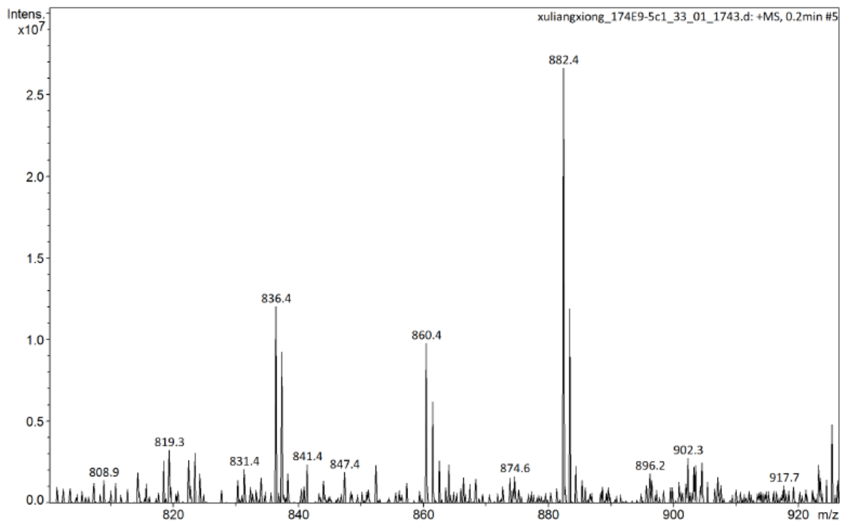
图 S12 化合物 1 的(+)-ESI-MS 谱
