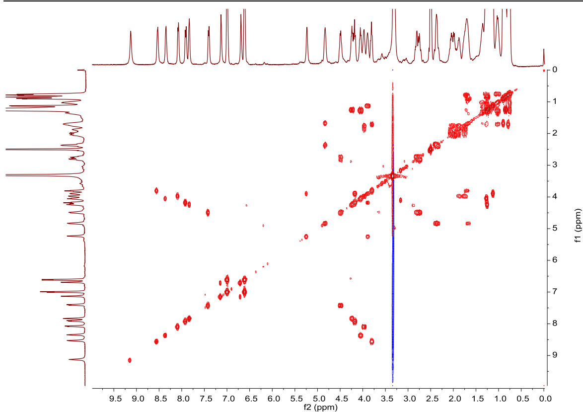
图 S3 化合物 1 的 ^1\text{H} - ^1\text{H} COSY 谱 (DMSO- d_6 )
