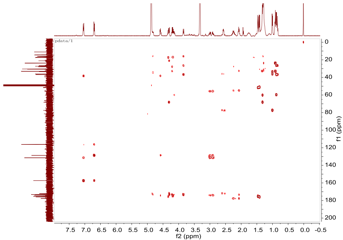
图 S10 化合物 1 的 HMBC 谱 (CD 3 OD)
