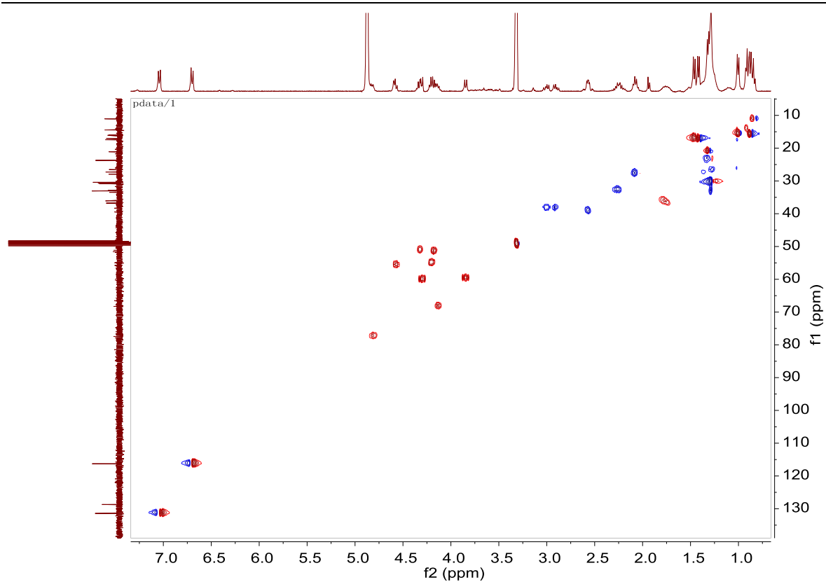
图 S9 化合物 1 的 HSQC 谱 (CD 3 OD)
