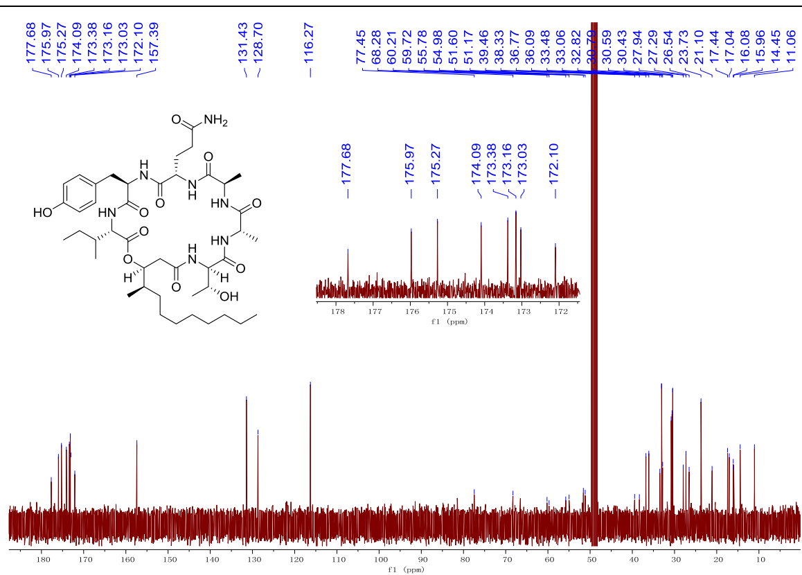
图 S7 化合物 1 的 ^{13}\text{C} NMR 谱 ( \text{CD}_3\text{OD} ) Figure S7. ^{13}\text{C} NMR spectrum of 1 in \text{CD}_3\text{OD}
