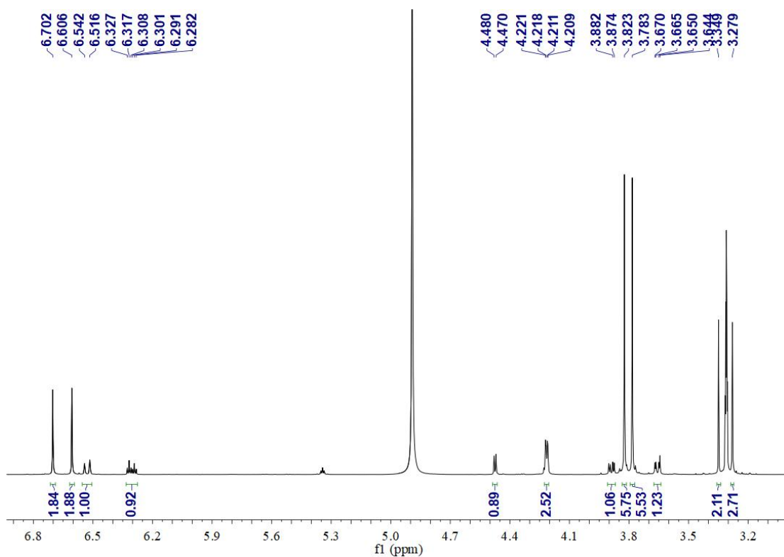
图 2 化合物 1 的 1 H NMR (600 MHz, CD 3 OD) 图谱
