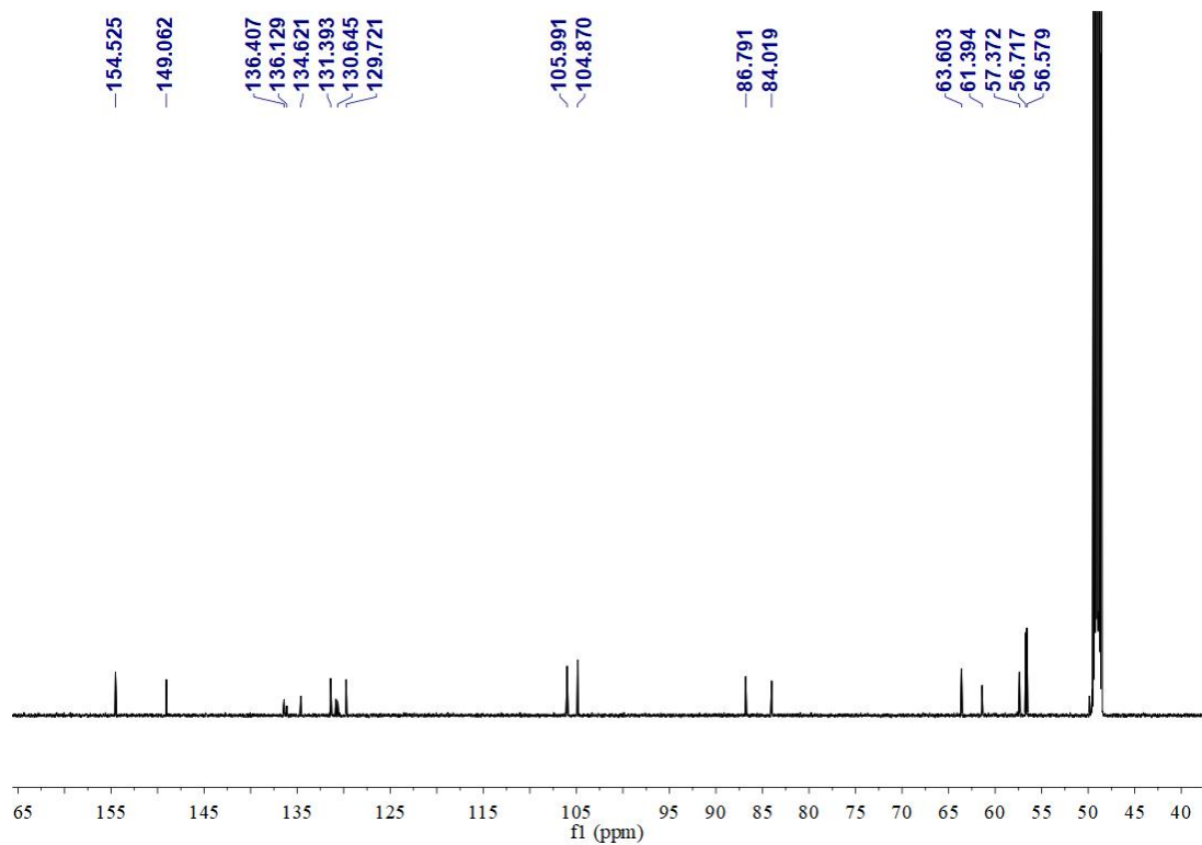
图3 化合物 1 的 ^{13}\text{C} NMR (150 MHz, \text{CD}_3\text{OD} ) 图谱
