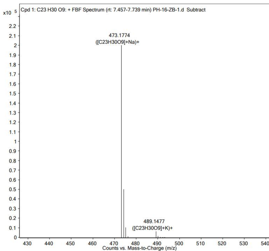
图 1 化合物 1 的 (+) HR-ESI-MS 图谱
