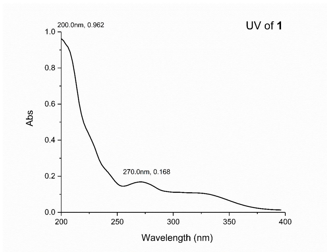
图 8 化合物 1 的 UV 图谱
