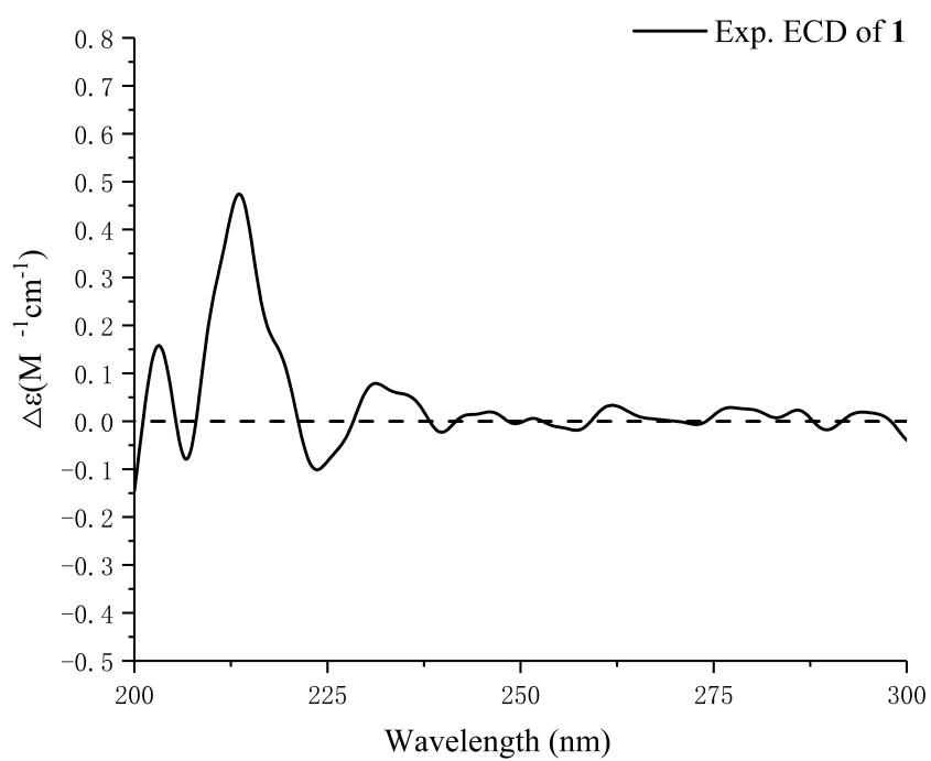
图 7 化合物 1 的 ECD 图谱
